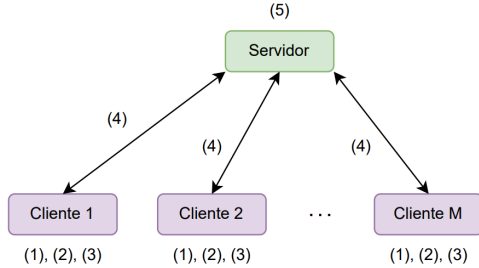
Fig. 1. Solución propuesta basada en OpenMax para escenarios de aprendizaje federado.
