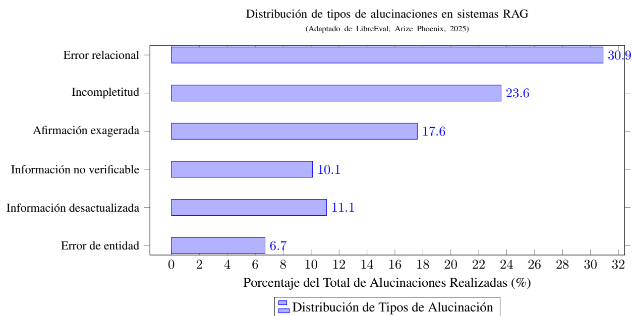
Figure 6: Distribución porcentual de los diferentes tipos de alucinaciones efectivamente realizadas en las respuestas de modelos de lenguaje con RAG, según el dataset LibreEval1.0. Esta distribución destaca los desafíos más comunes que las estrategias de mitigación deben abordar.
