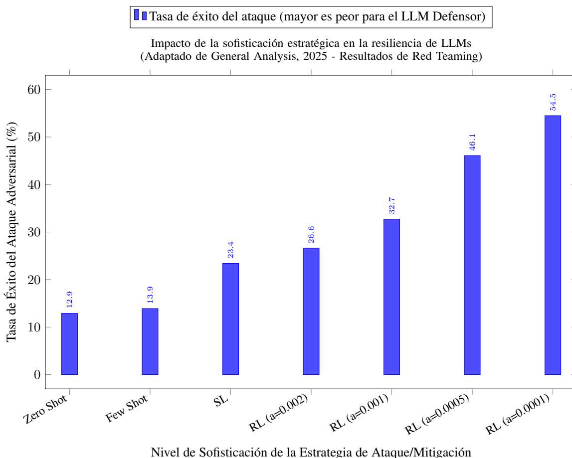
Figure 4: Esta gráfica ilustra cómo estrategias de ataque más sofisticadas (análogas a la falta de estrategias de mitigación robustas o a vulnerabilidades explotadas) logran una mayor tasa de éxito al inducir fallos en un LLM objetivo (GPT-4o). Demuestra la necesidad de estrategias de defensa (mitigación) igualmente sofisticadas. El eje X representa diferentes algoritmos de ataque del estudio de General Analysis, interpretados aquí como niveles de desafío o sofisticación a los que un sistema RAG legal debe ser resiliente.
