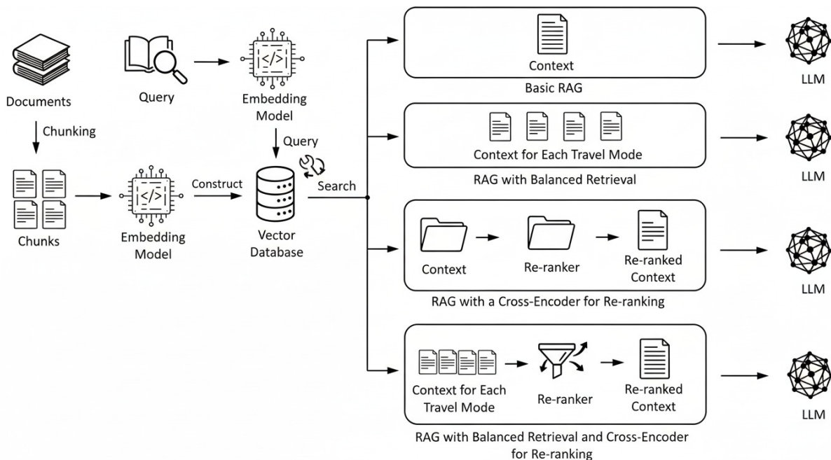
Figure 3: Diagrama esquemático de un sistema de generación aumentada por recuperación (RAG). El flujo ilustra cómo una consulta de usuario (Input Query) se enriquece con información contextual recuperada de una base de conocimiento externa (Vectorstore) antes de ser enviada al LLM. Este proceso ancla la respuesta en datos verificables, mitigando la generación de alucinaciones. Adaptado de Yiming Xu et al. (2025).
