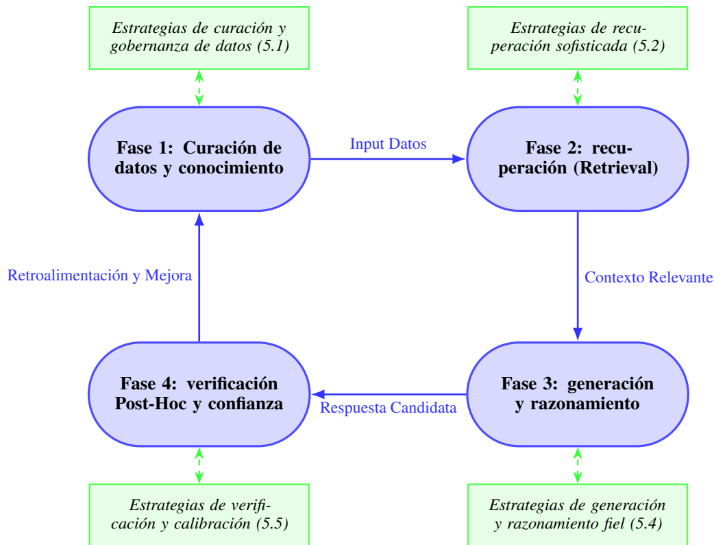
Figure 5: Modelo cíclico de un sistema RAG Legal y puntos de intervención estratégica para la optimización y mitigación de alucinaciones. Las estrategias específicas (referenciadas por subsección del ensayo) se aplican en cada fase para mejorar la fiabilidad general del sistema.
